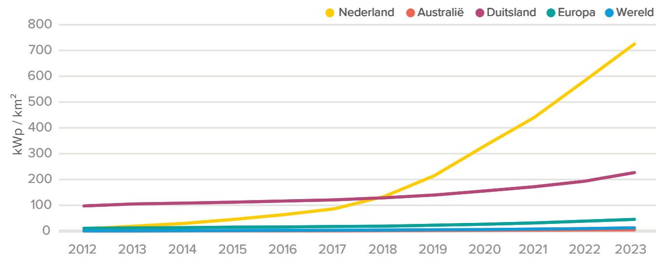
Zonnestroomvermogen per vierkante kilometer 5,6,7,8,9 (Fig. 6)
